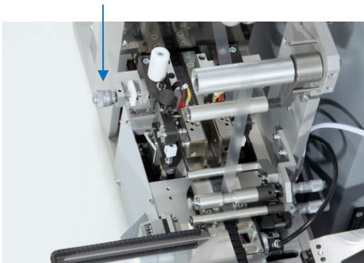
Schweißkufen mit Mikrometerschraube
