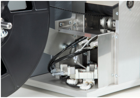
Gurtvorschub mit Schrittmotor
